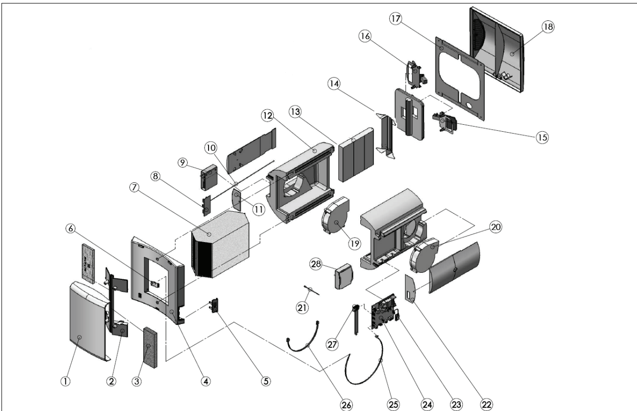
Abb. 2.4 Geräteaufbau im Detail
